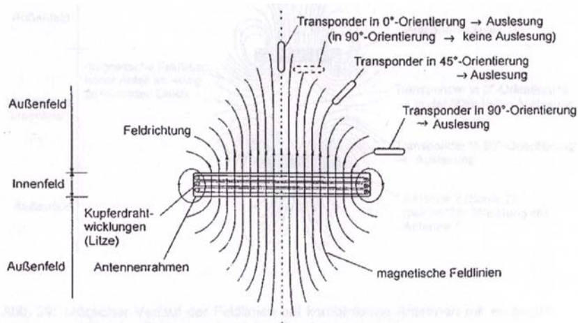
Abbildung 2: Feldlinienverläufe bei einer Einzelantenne und die Auswirkung auf die Transponderlesung Quelle: KERN 1997
