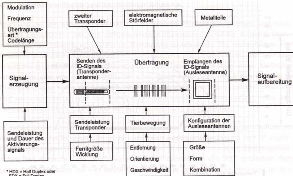
Abbildung 3: Einflussfaktoren auf die Übertragung des Erkennungssignals bei Transpondern am Beispiel des Injektats Quelle: PIRKELMANN, KERN (1994)
